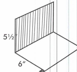
ENDWALL
