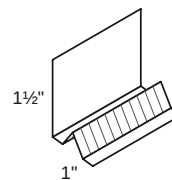
Header face
